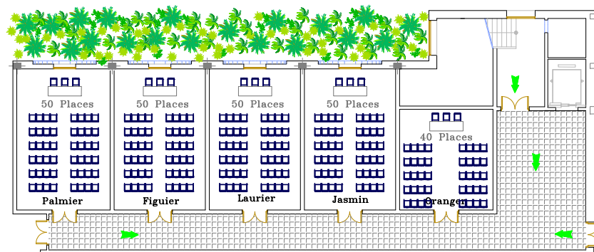
PLAN SALLE DE SOUS COMMISSION ( NIVEAU REZ DE CHAUSSÉE )
